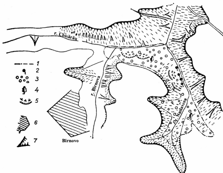
Sectorul natural "La cele 33 de vaduri". Schita topografică.
